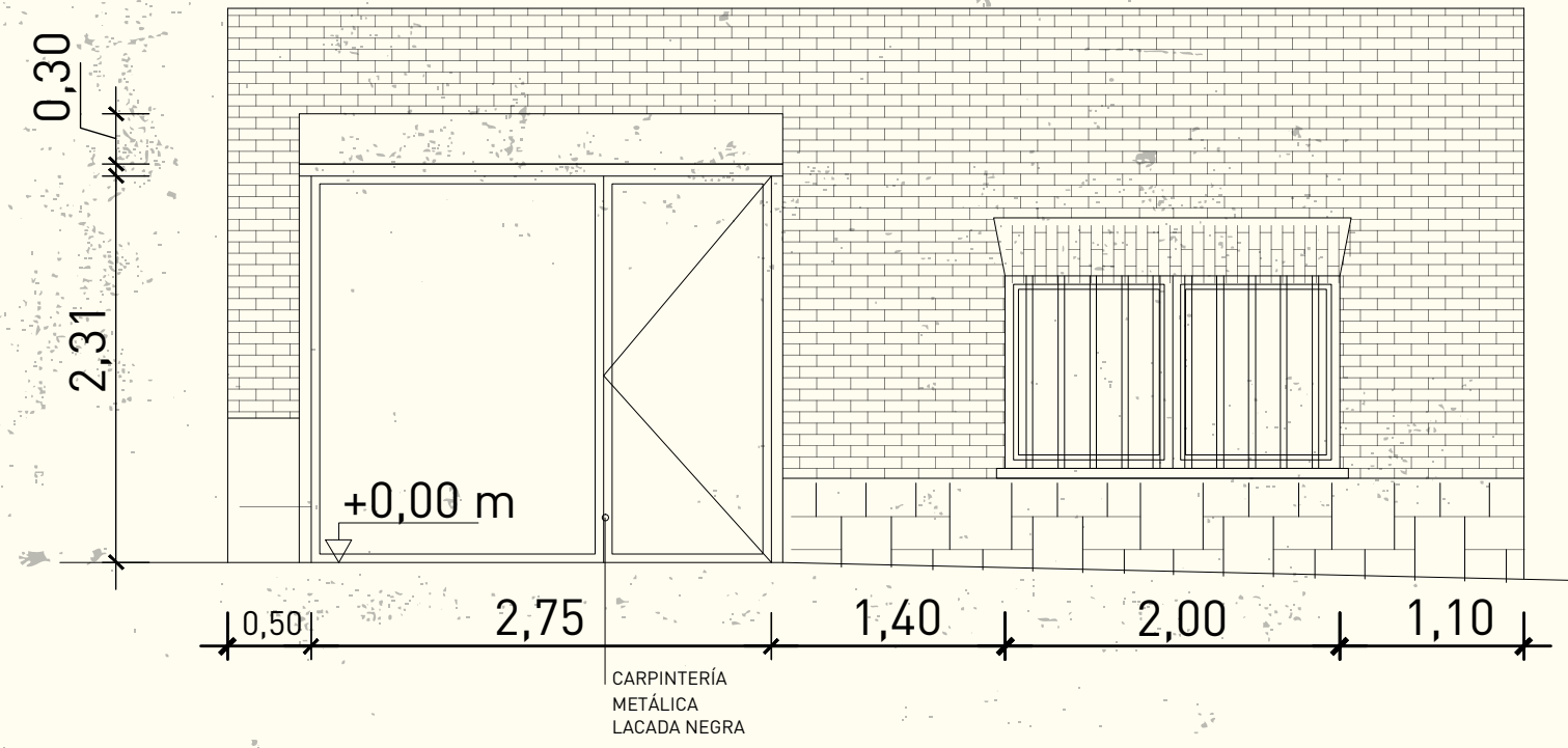
ALZADO 1
